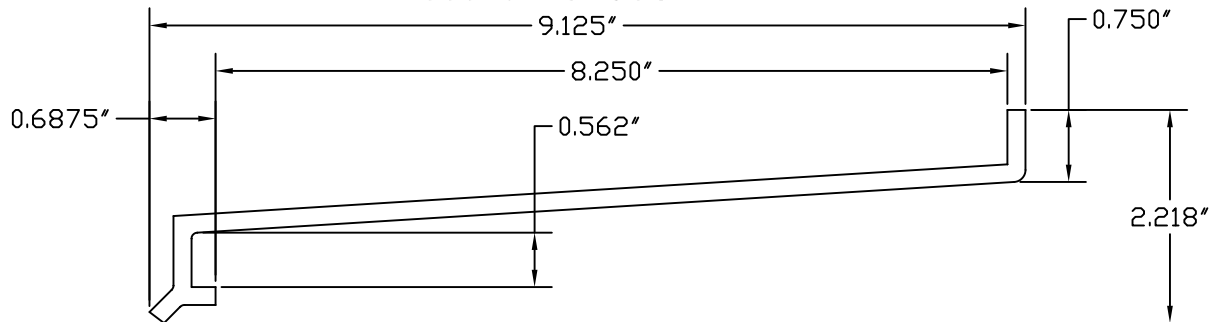
Alcoa Sill 54693
